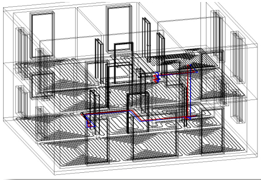
IVT-Planungsleistung Ansicht Flächenheizung
